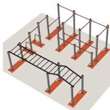
ID Товара 4306 Габариты: 5,5x4,9x2,2 Материал: Сталь, труба 102, хомуты
